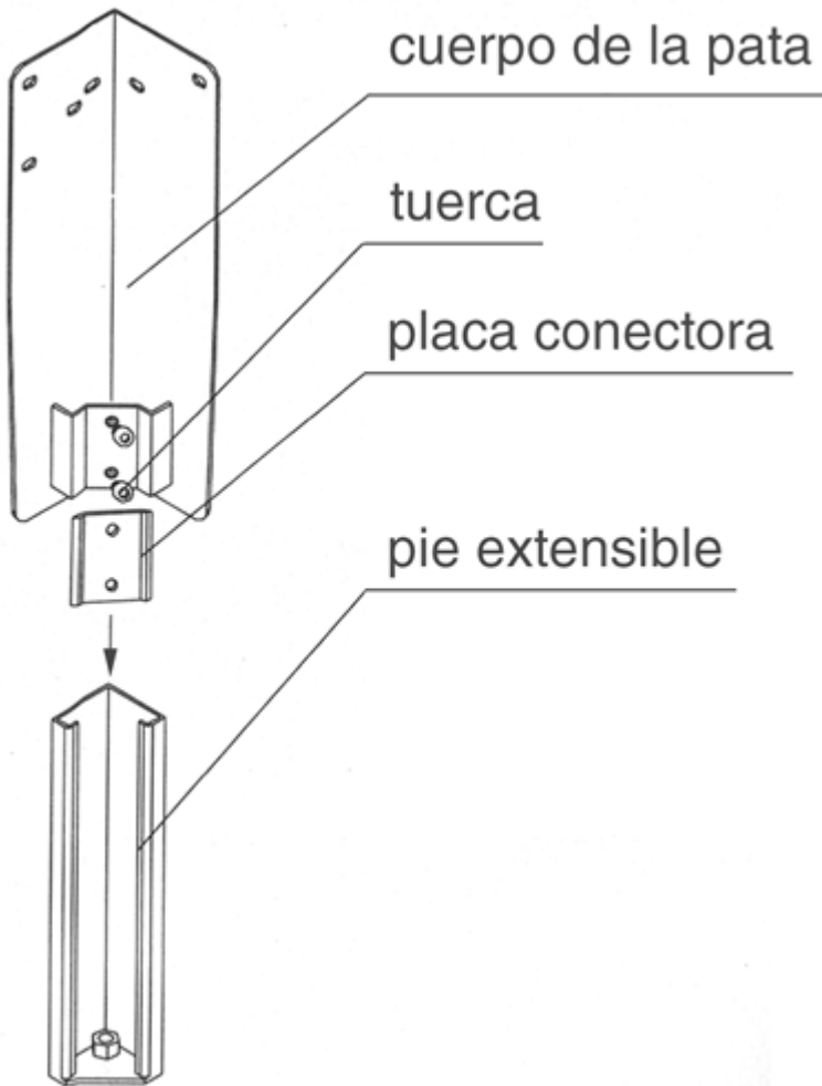
Esquema precintadora
